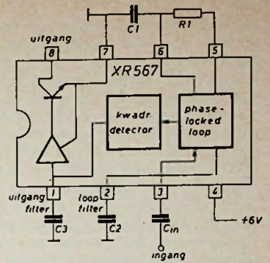
Fig. 2. Functieschema van de XR-567.
